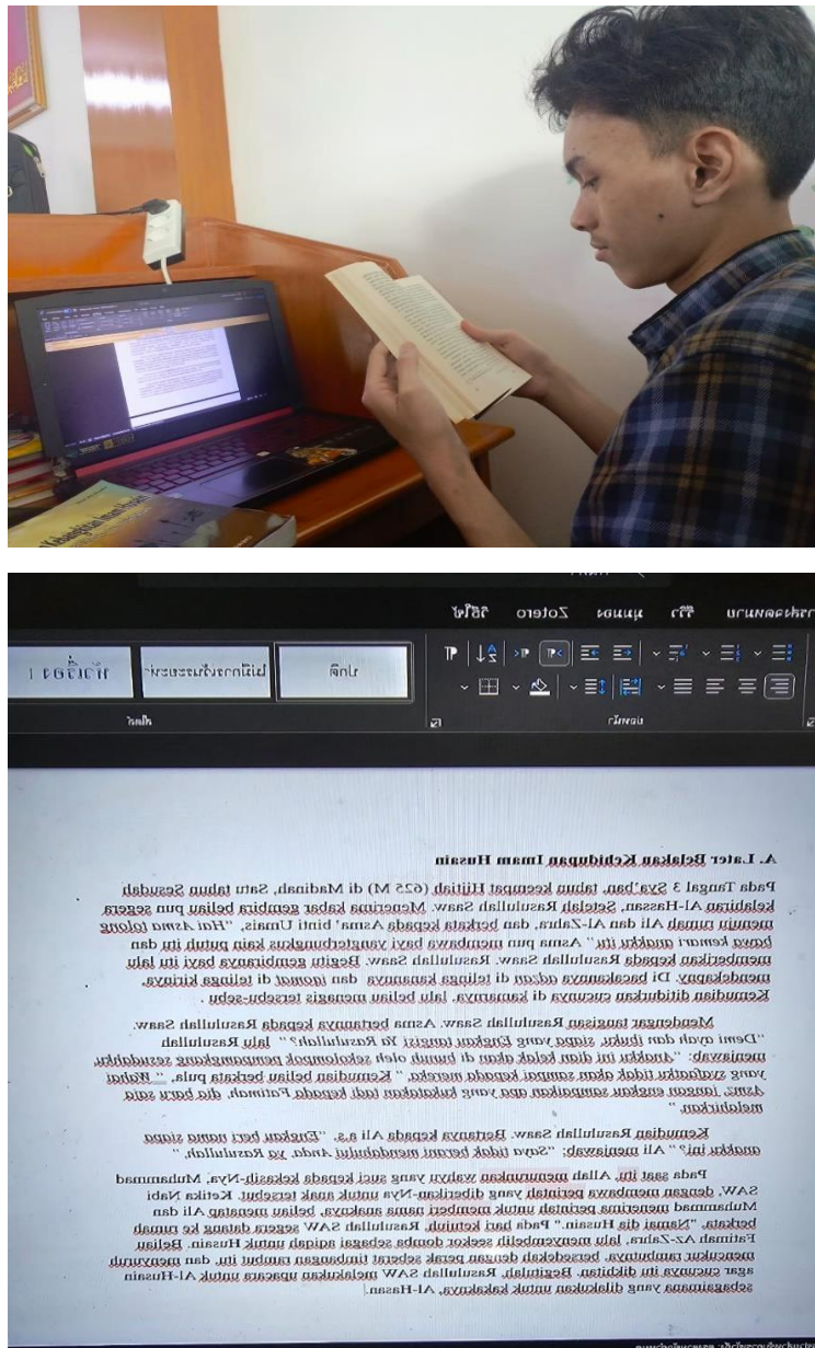
Gambar 3.4 Membuat Artikel
